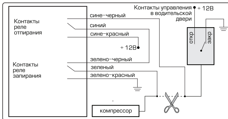
Схема подключения к пневматической системе запирания
